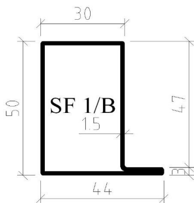
1. PROFIL Z ENOJNO PRIPIRO
